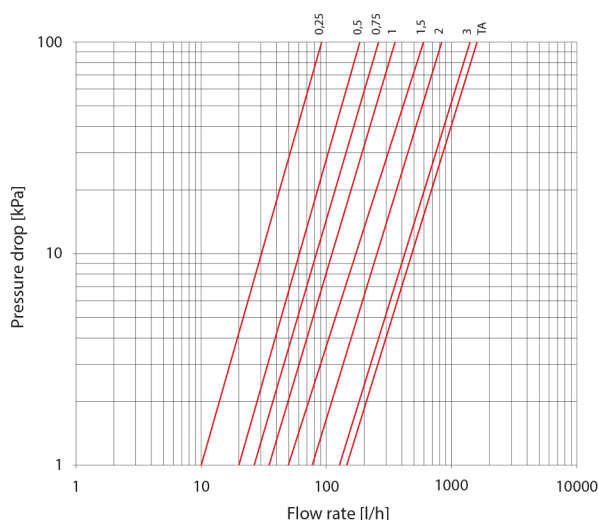
Diagramme du détendeur de réglage (collecteur de départ)
