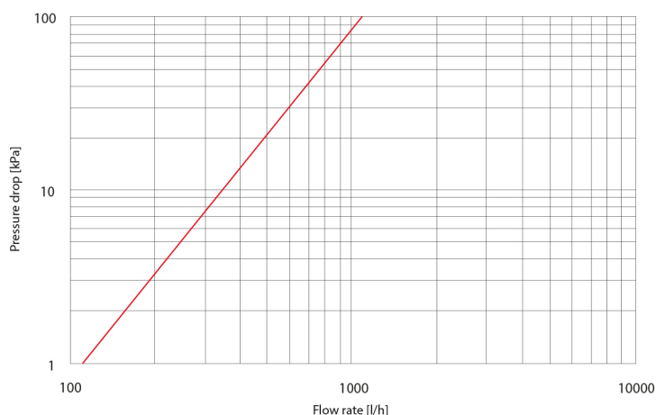
Diagramme débitmètre totalement ouvert (collecteur de départ)
