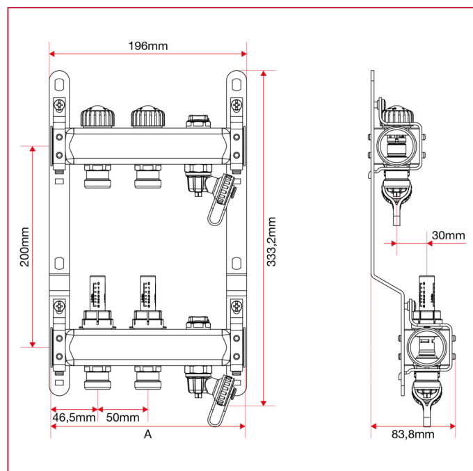
型号 91780CDEB 总尺寸
