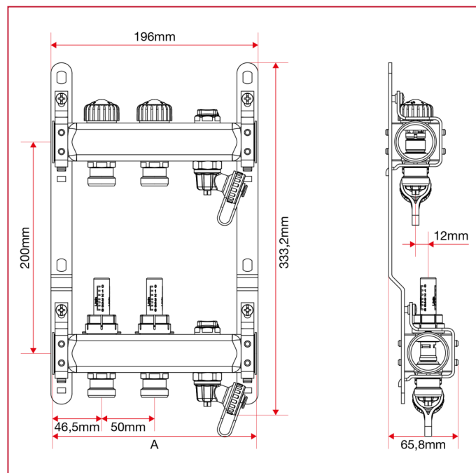
型号 917CDEB 总尺寸
