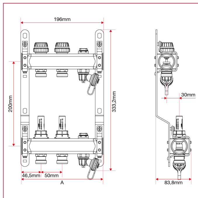
型号 91780CDE 总尺寸
