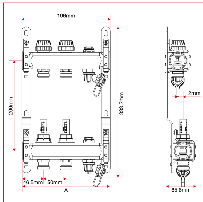
型号 917CDE 总尺寸
