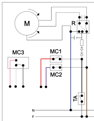
计时器 (CO - HC) 环境温控器 (TA - ET) 电源连接图 计数通过计时器实现，计算阀打开的总时间。 该图显示了无计时器的执行器电气连接。
