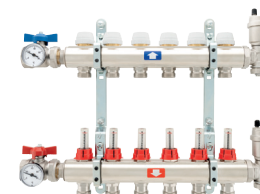
COLLETTORI PREMONTATI OTTONE
