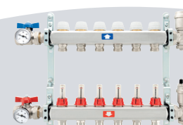
COLLETTORI PREMONTATI INOX
